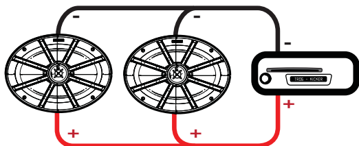
Zwei PS-Lautsprecher parallel mit einem einzelnen Kanal verdrahtet
